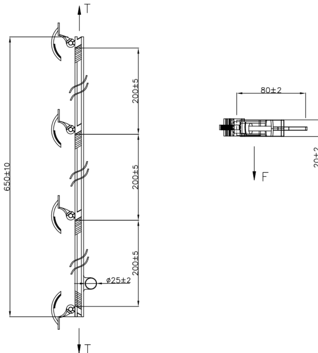
Figura 2 - Espaçador para 4 Cabos - Tipo 2
