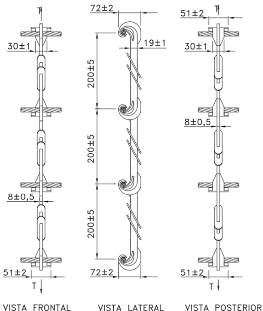
Figura 1 – Espaçador para 4 Cabos – Tipo 1
