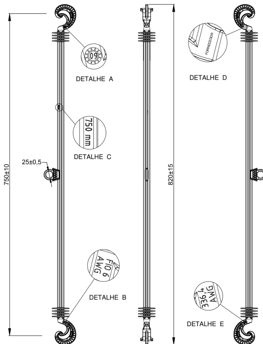
Figura 3 - Espaçador horizontal para redes primárias - tipo 3
